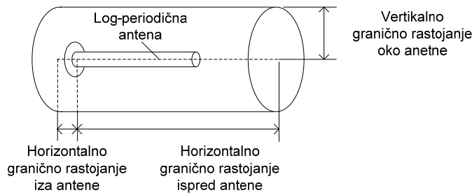
Slika 3. Zona nedozvoljenog zračenja za log-periodičnu antenu
