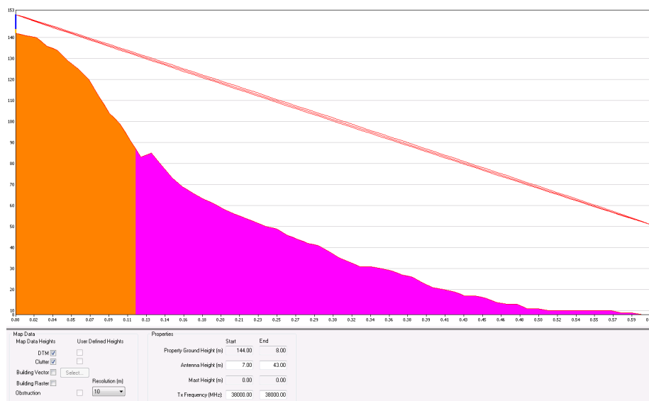
Skica: Profil trase Sušćepan - Hotel Metalurg (Lighthouse) (sa ucrtanom I - Frenelovom zonom)
