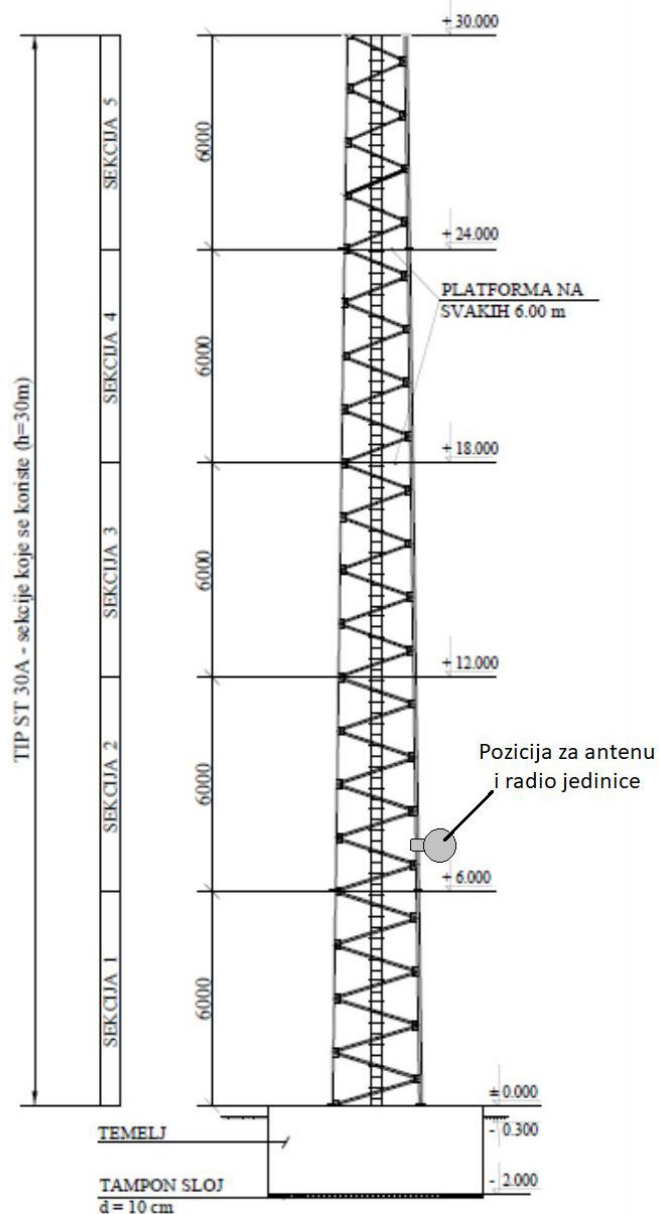
Skica: Pozicija za antenu i radio jedinicu (Antena i radio jedinice se montiraju na nogu stuba u pojasu 7m)
